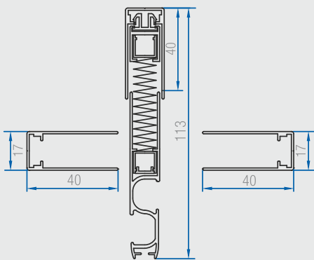
Inset Mount / İçe Montaj
