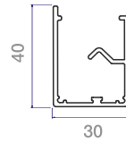
Top guide 30x40
