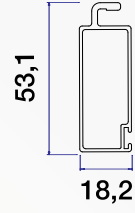
Kanat Profil 18,2x53,1
