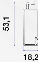
Kanat profil 18,2x53,1
