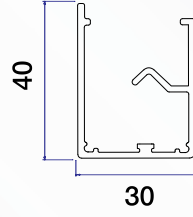
Üst Profil 30x40
