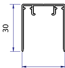
Upper guide
