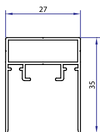
Top guide
