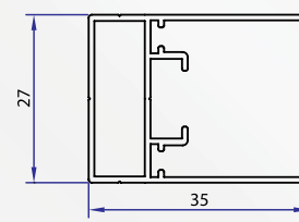
Side guide
