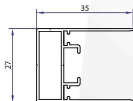
Side guide
