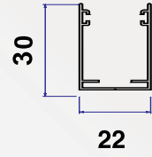
30 x 22 mm Dikme
