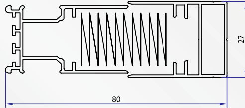
TÜL Gövdesi
