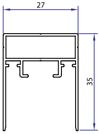
Üst Klavuz
