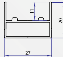
Alt Klavuz
