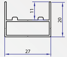
Alt Klavuz
