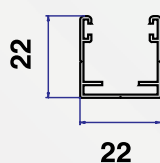
Guide low 22x22
